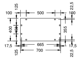
TABAN DELİK ÖLÇÜSÜ BOTTOM HOLE SIZE
