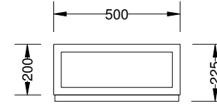
ÜST GÖRÜNÜŞ TOP VIEW
