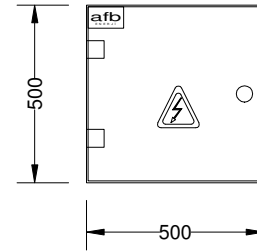
KAPAKLI ÖN GÖRÜNÜŞ FRONT VIEW WITH DOOR
