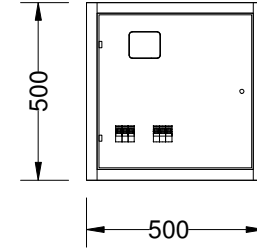
İÇ GÖĞÜS KAPALI ÖN GÖRÜNÜŞ FRONT VIEW WITH INTERIOR DOOR
